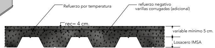
SECCION A-A
